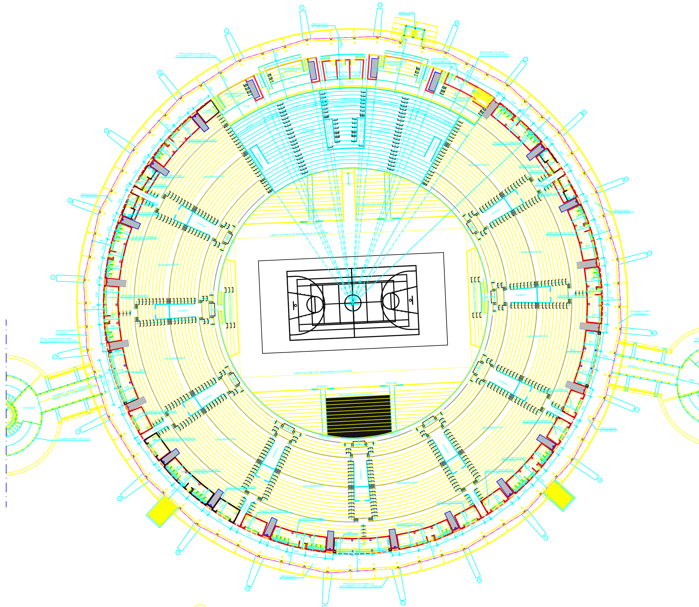
1 PLANTA BAIXA - 4º PAV ESC.: 1/250
